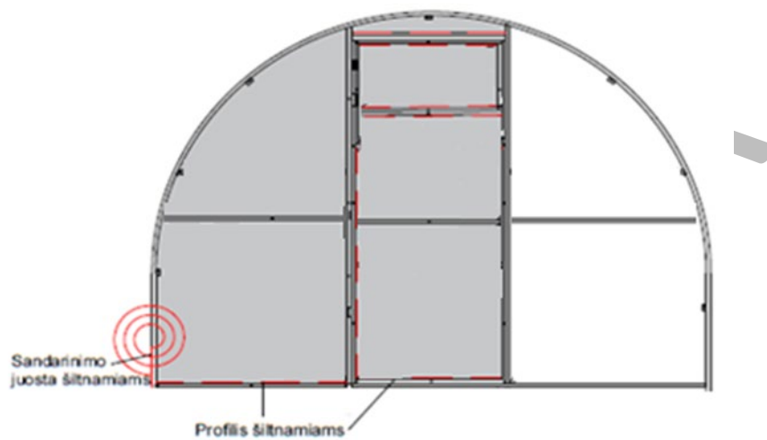
Pav. 5 Polikarbonato dangos montavimas ant šiltnamio rėmo
