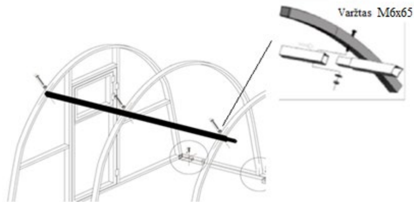
Pav. 12. Tvirtinimas naudojant suveržiamąsias templates
