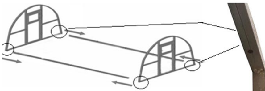
Pav.8. Šiltnamio priekinės ir galinės arkos tvirtinimas
