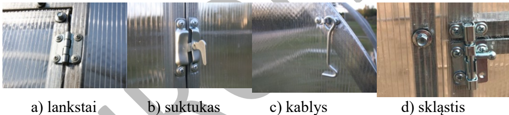
Pav. 16 Suktukų, skląsčių, lankstų, kabliukų tvirtinimo vietos ant šiltnamio arkos
