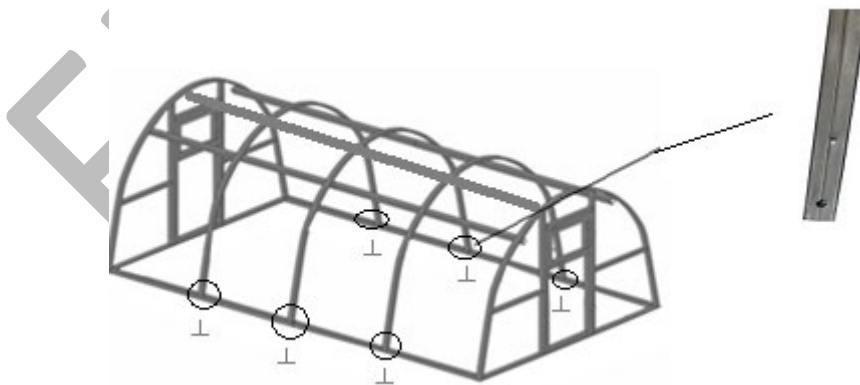
Pav. 11. Lankų tvirtinimas
